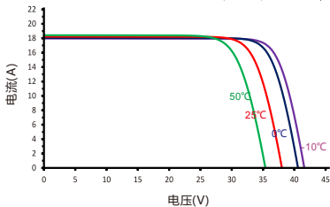
不同电池温度下, I-V 曲线图
