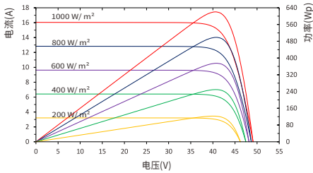
RSM132-11-620BNDG 不同辐照度下, I-V 曲线图
