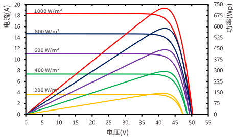
RSM132-8-730BHDG 不同辐照度下, I-V 曲线图
